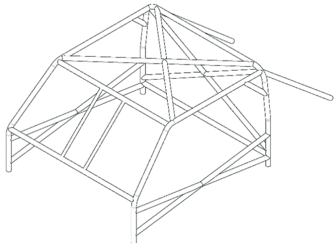
Tekening 2) Rolkooi optie 2
